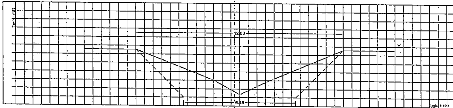
STA 0+350
