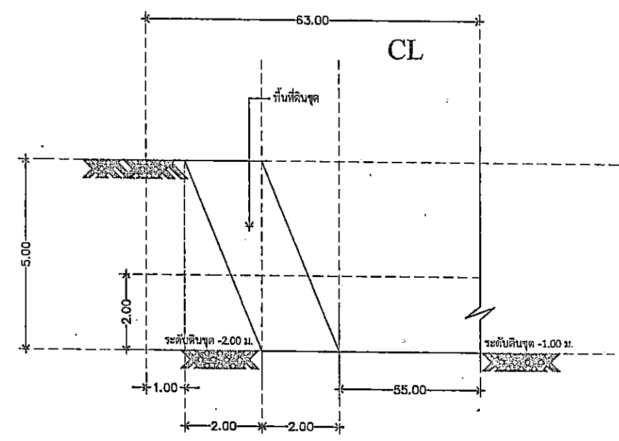
รูปตัด B - B SCALE N. T. S.
