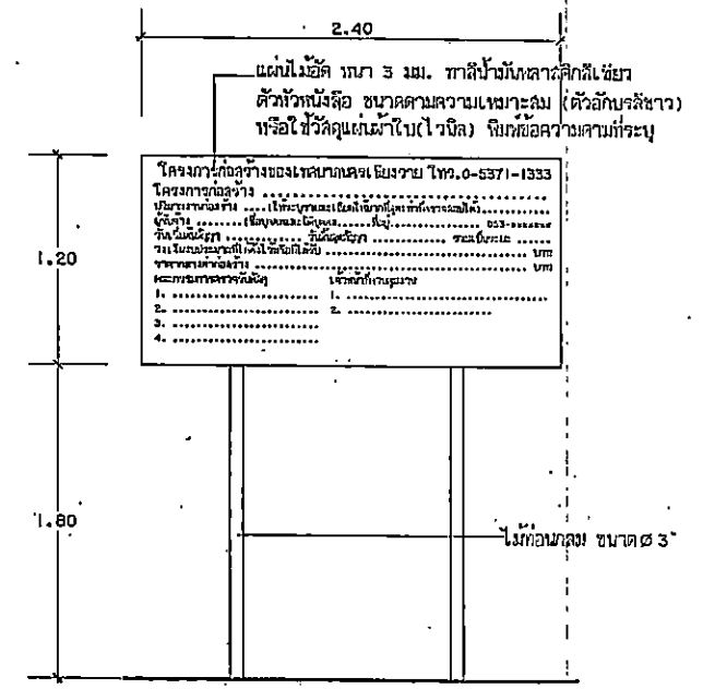
แบบป้ายประชาสัมพันธ์ระหว่างอาคารก่อสร้าง
