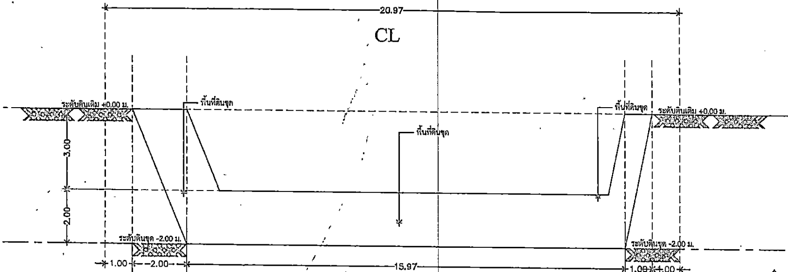
รูปตัด C - C SCALE 1 : 100
