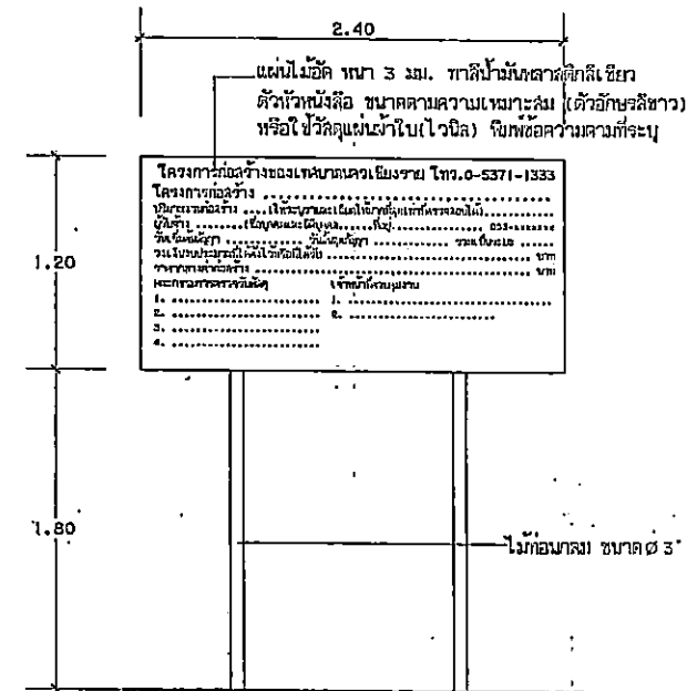
แบบป้ายประชาสัมพันธ์ระหว่างการก่อสร้าง
