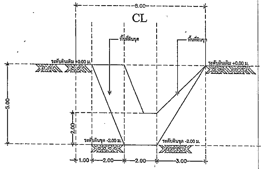
รูปตัด A - A SCALE 1 : 100
