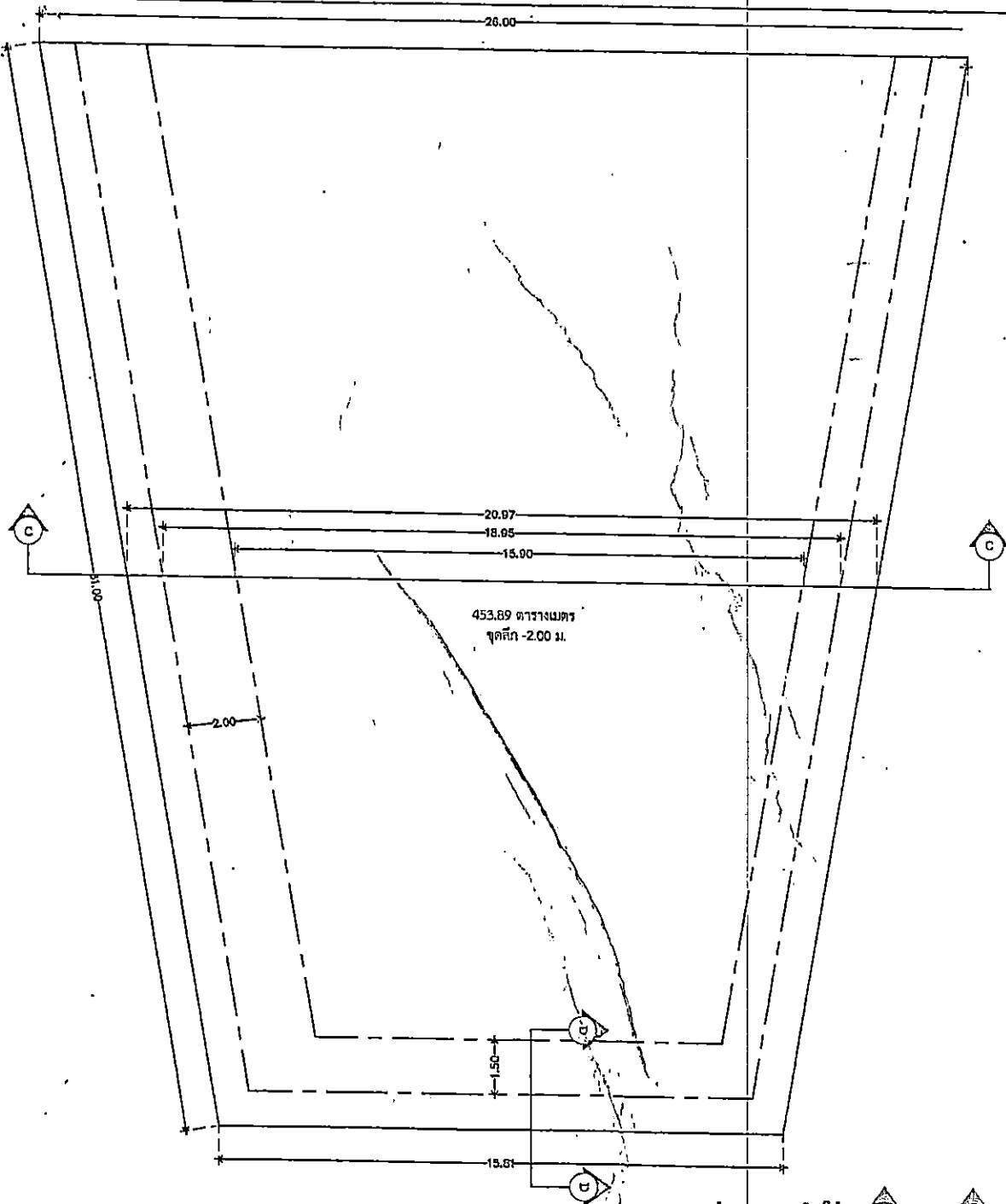
แปลนรูปตัด C - C และ D - D SCALE N. T. S.
