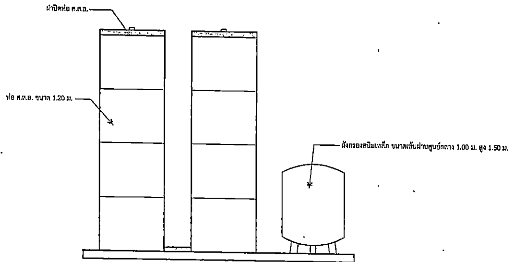
รูปด้านข้าง Scale 1:50
