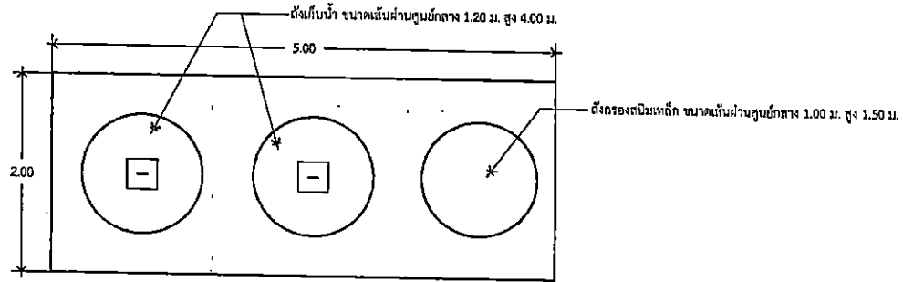
แปลน Scale 1:50
