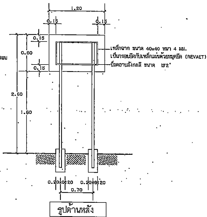
แบบป้ายประชาสัมพันธ์ระหว่างอาคารก่อสร้าง
