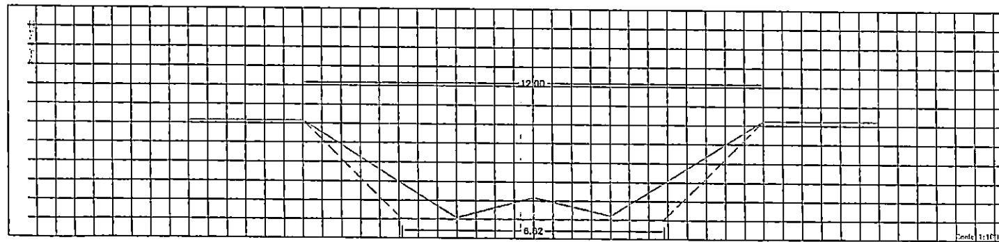
STA 0+550
