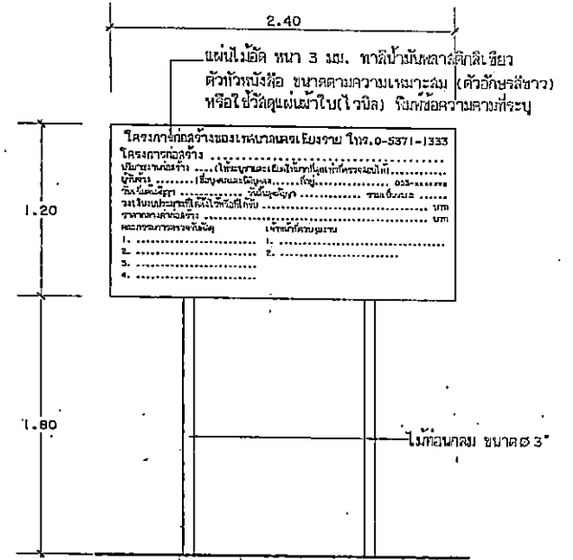
แบบป้ายประชาสัมพันธ์พื้นที่ระหว่างอาคารก่อสร้าง
